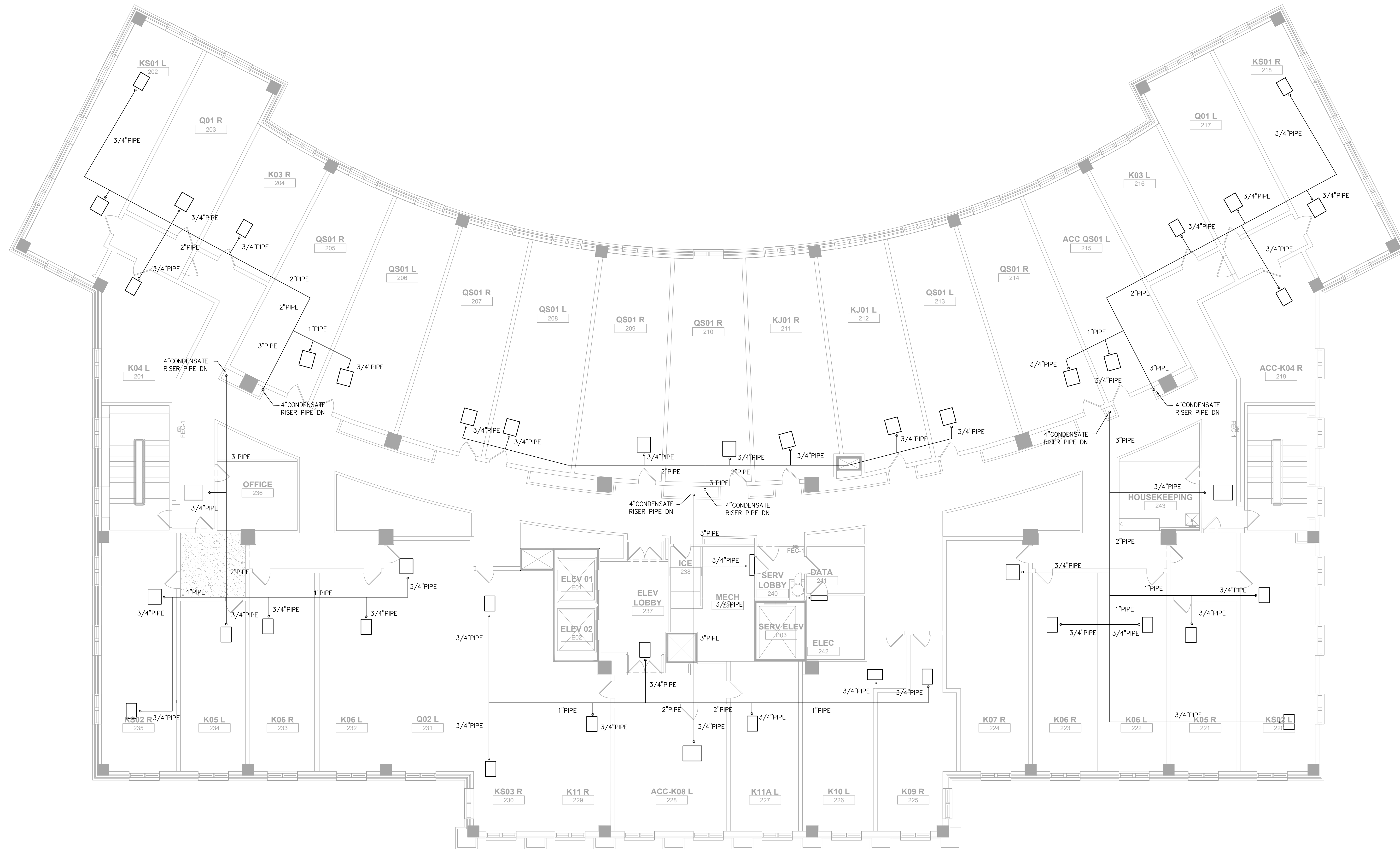
1 Plumbing Condensate Floor Plan - Level 2 Scale: 1/8" = 1'0"
