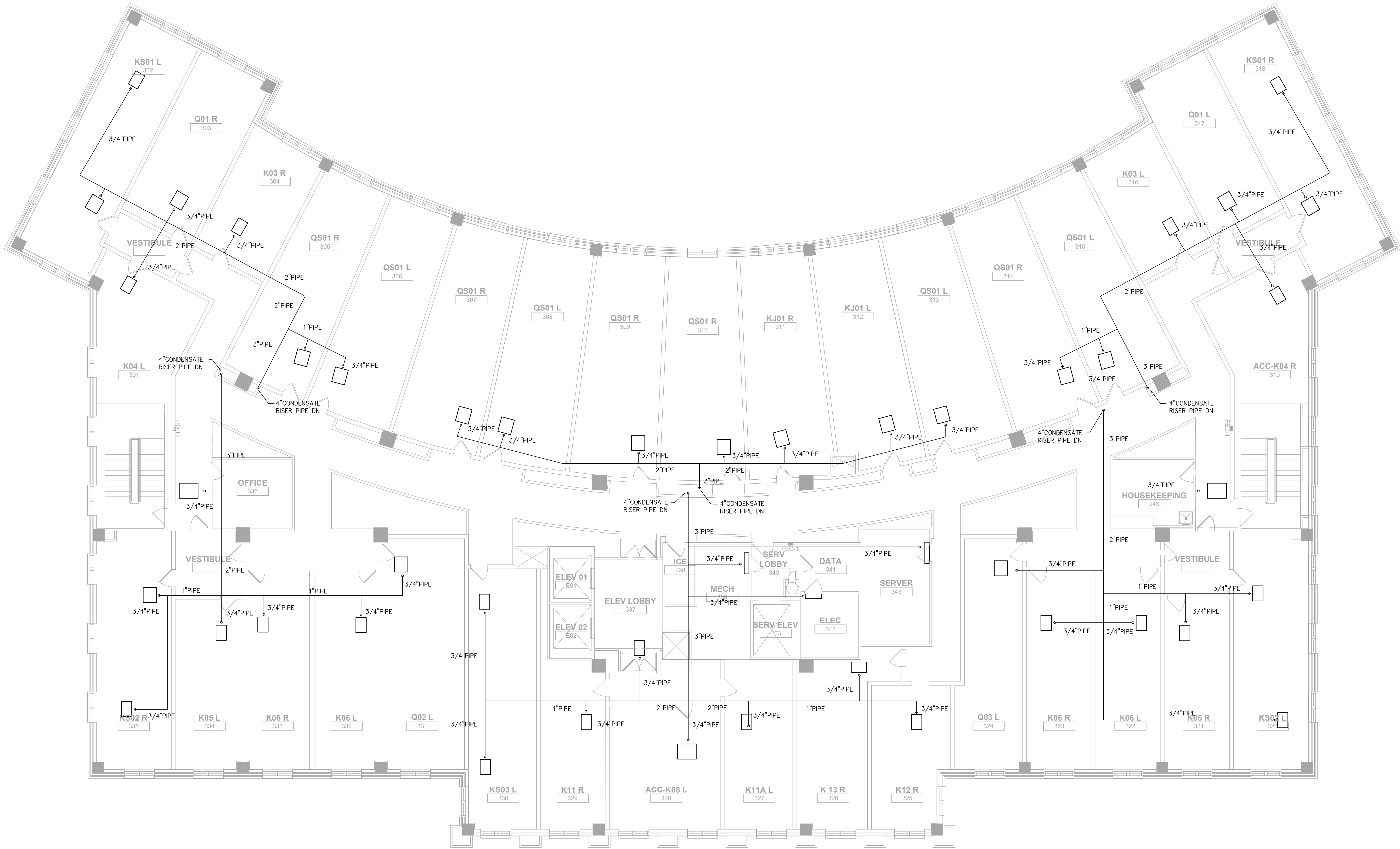
1 Plumbing Condensate Floor Plan - Level 3 Scale: 1/8" = 1'-0"
