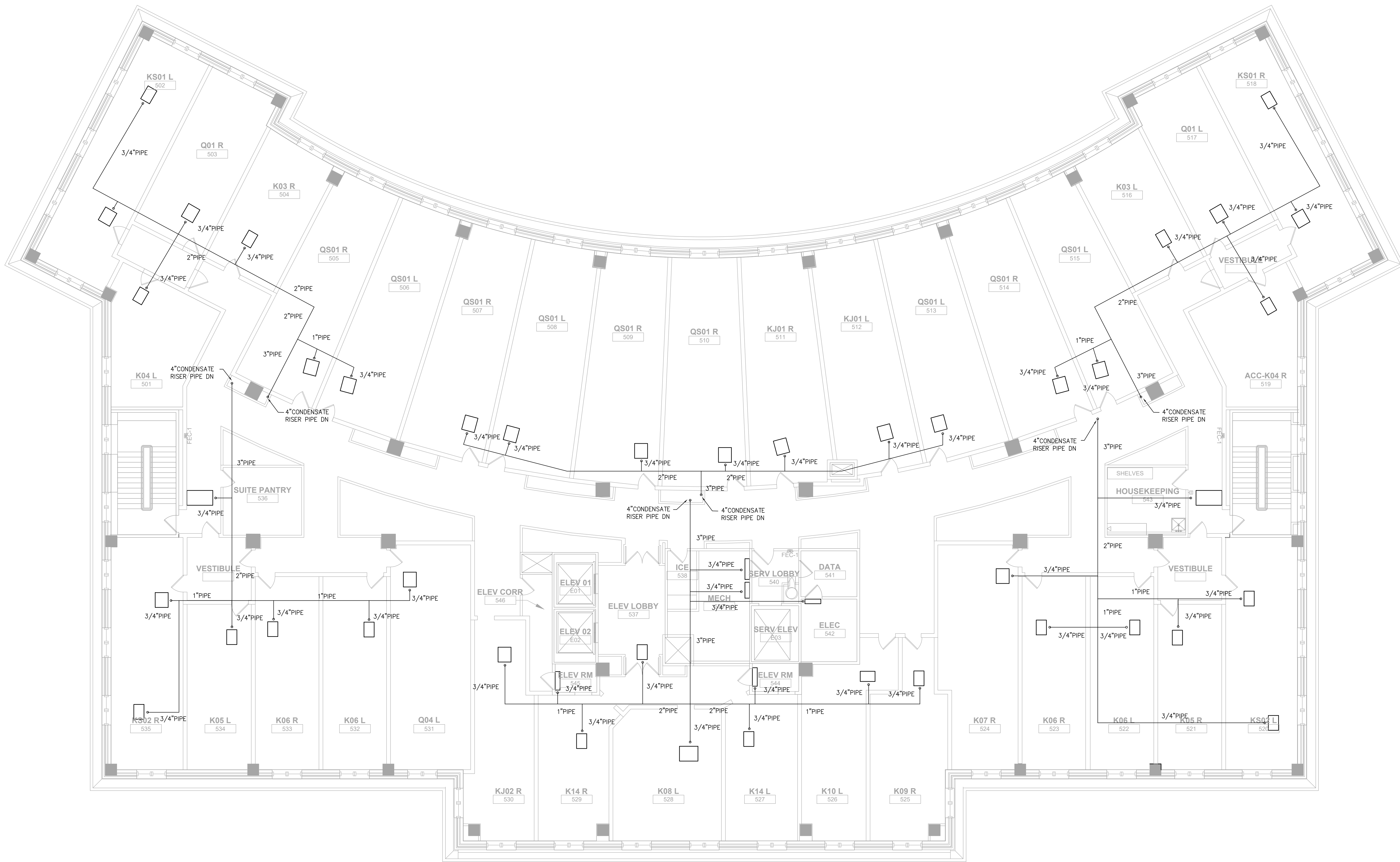
1 Plumbing Condensate Floor Plan - Level 5 Scale: 1/8" = 1'0"
